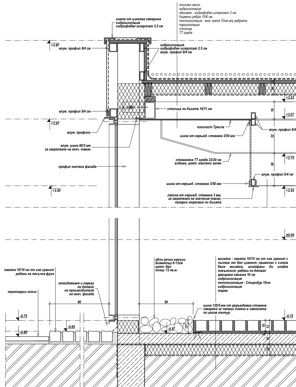
Детайлен разрез Р-03 М 1:10
