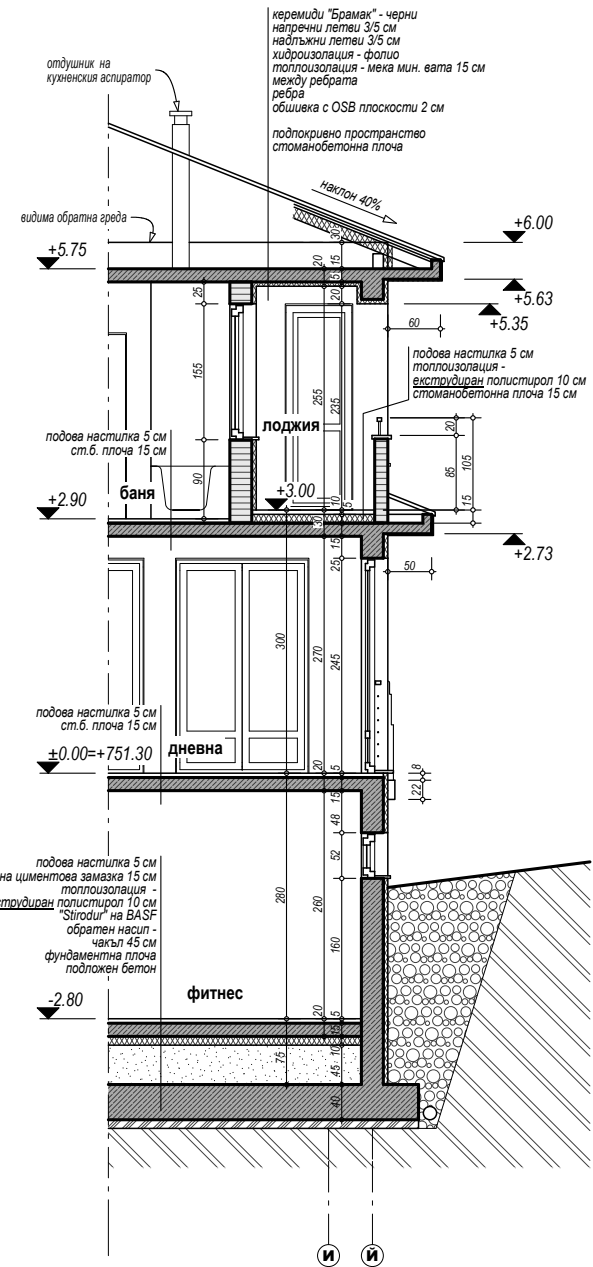
Разрез 4-4
